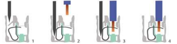
Yaylı Bağlantı
