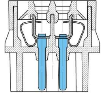
Yaylı Bağlantı
