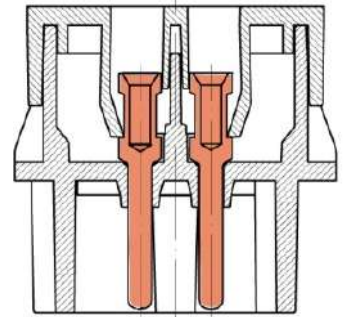
Krimp Bağlantı
