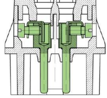
Vidalı Bağlantı
